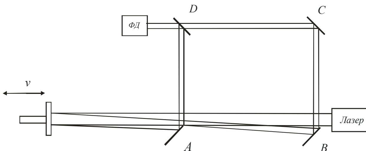
Рис. 4. Схема интерферометра с отражательным зеркалом.
