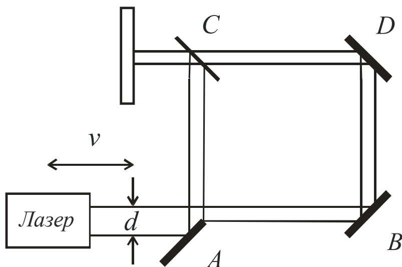
Рис. 3. Схема интерферометра с механическим делением луча лазера
